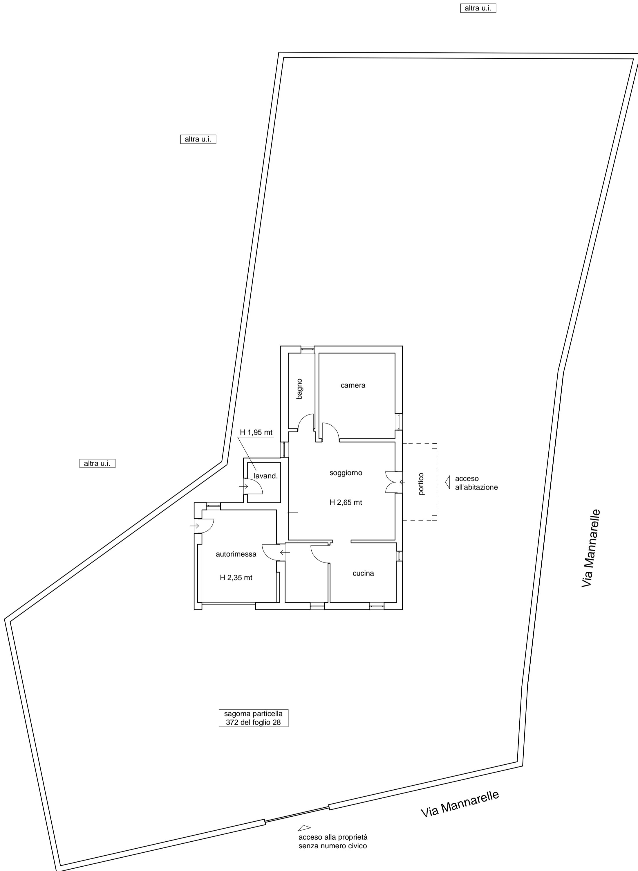
Pianta Piano Terra Scala 1:100
